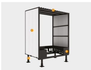
ABRI NIVELEUR
