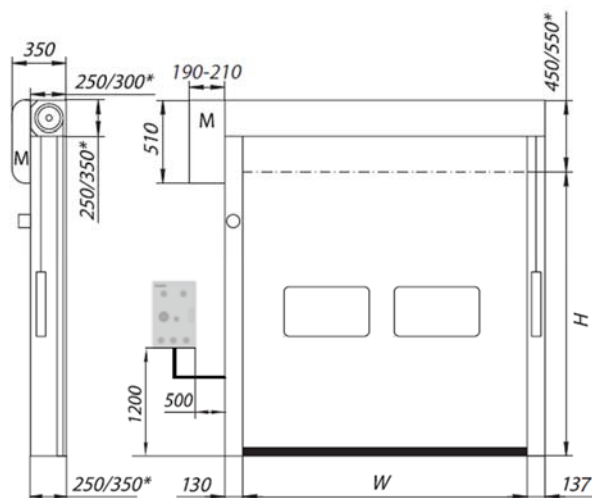
Moteur en position latérale
