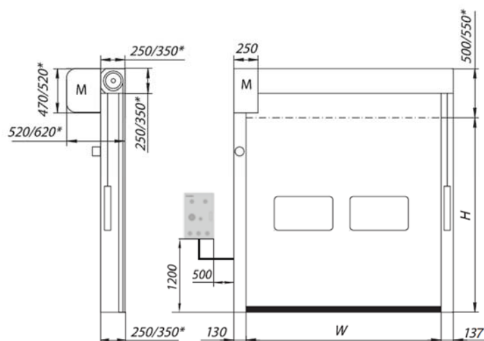
Moteur en position frontale
