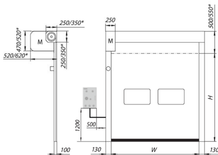
Moteur en position latérale avec contre-poids
