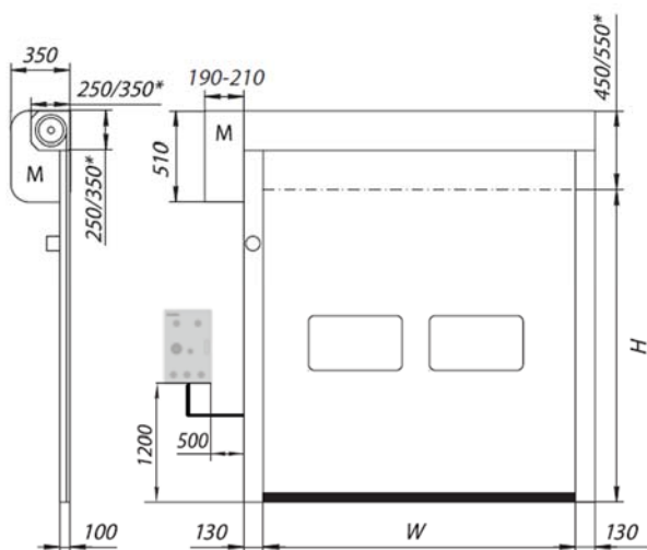
Moteur en position latérale avec contre-poids
